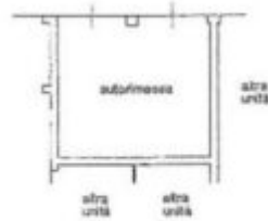
PIANO SOTTOSTRADA H.2250
